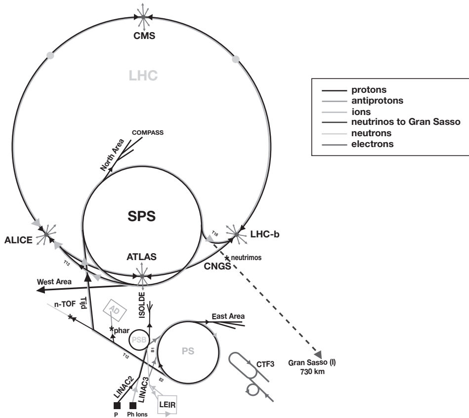
Figuur 1: Schematische voorstelling van het versnellercomplex van CERN
