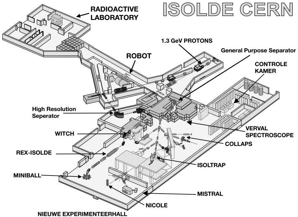
Figuur 10: Grondplan van de ISOLDE-opstelling
